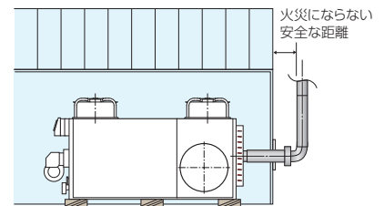
煙突真後出し例
