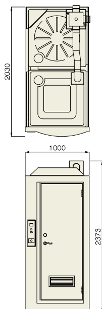
寸法図
