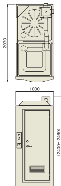
寸法図
