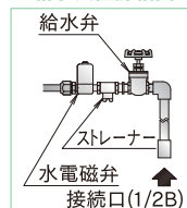
給水装置詳細図*
