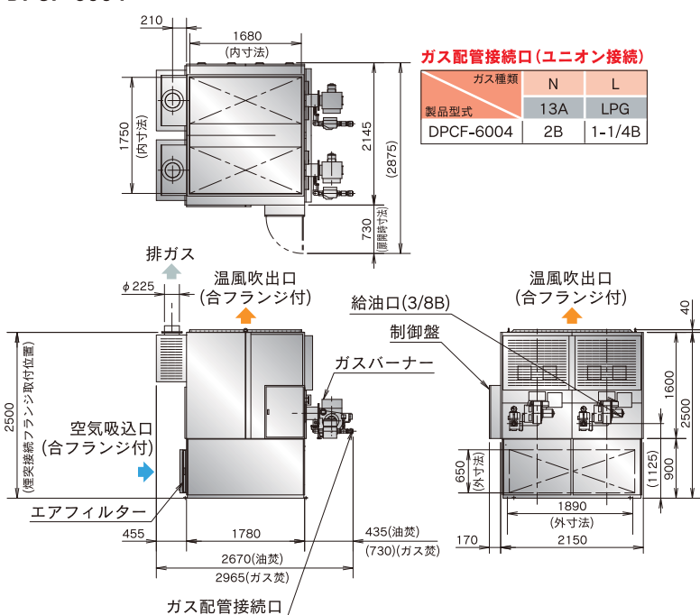
ガス配管接続口(ユニオン接続)
