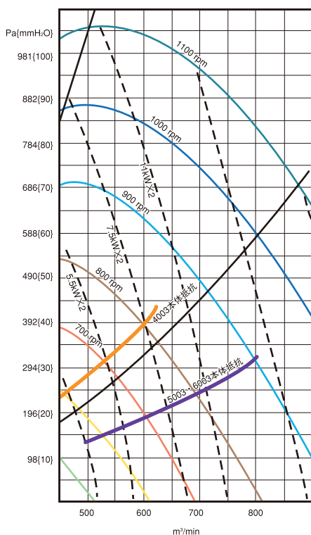
PCF-4003,5003,6003 送風機特性
