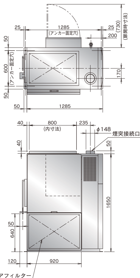
ガス配管接続口(ユニオン接続)
