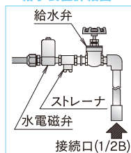
給水装置詳細図*
