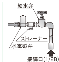
給水装置詳細図*
