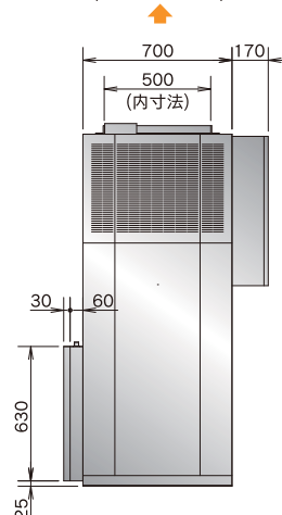
温風吹出口 (合フランジ付)
