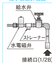
給水装置詳細図*
