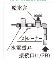
給水装置詳細図*
