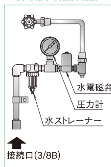
自動給水装置詳細図*
