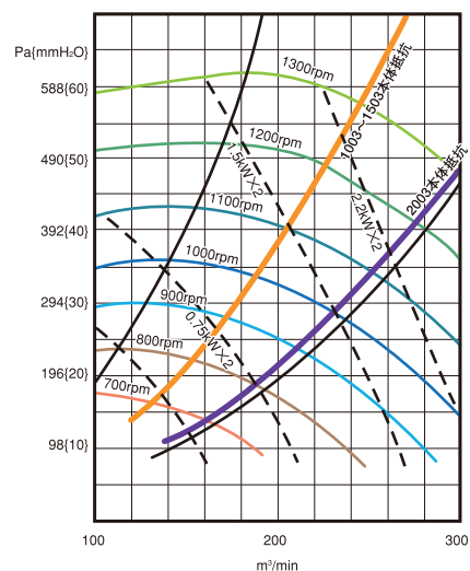
PFB-1003,1253, 1503,2003 送風機特性
