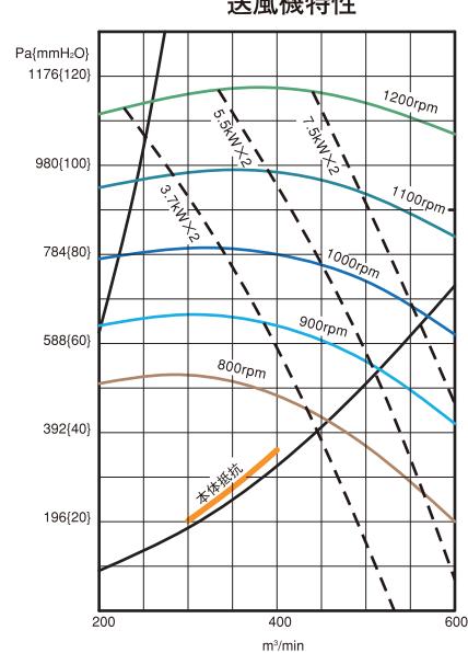
DPCF-6004 送風機特性
