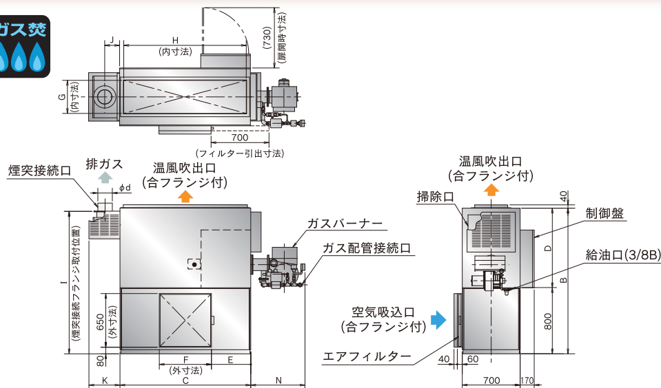
ガス配管接続口(ユニオン接続)
