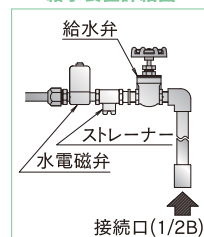
給水装置詳細図*
