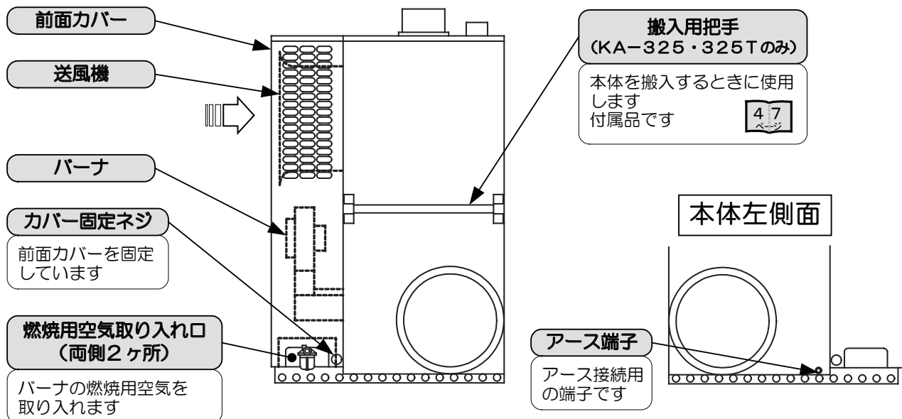
側面（例：KA-325）
