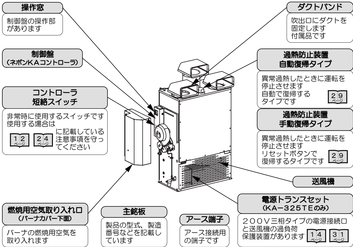
前面（例：KA-325E）
