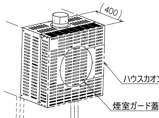
取付完成参考図
