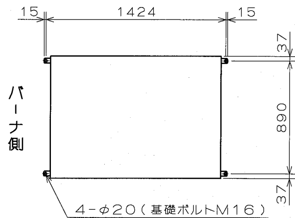
基礎ボルト固定位置 (S=1/30)
