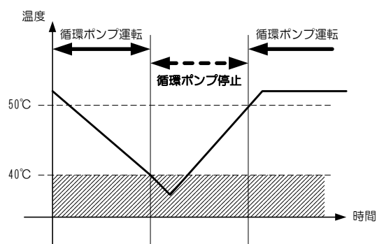
缶水温度の時間変化 (模式図)
