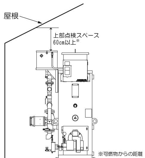
上部点検スペースの取り方
