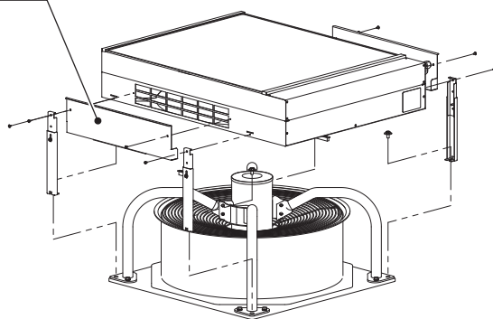
バイパスふさぎ板 (2枚)
