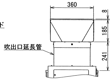
吹出口延長管取付参考図
