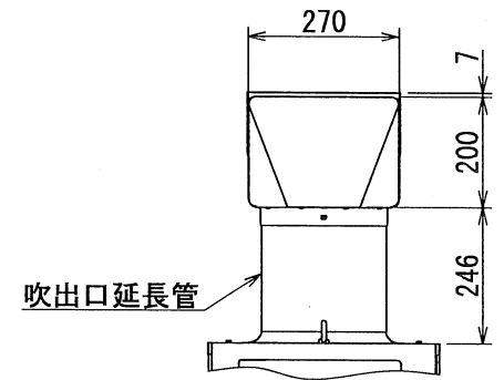
吹出口延長管取付参考図
