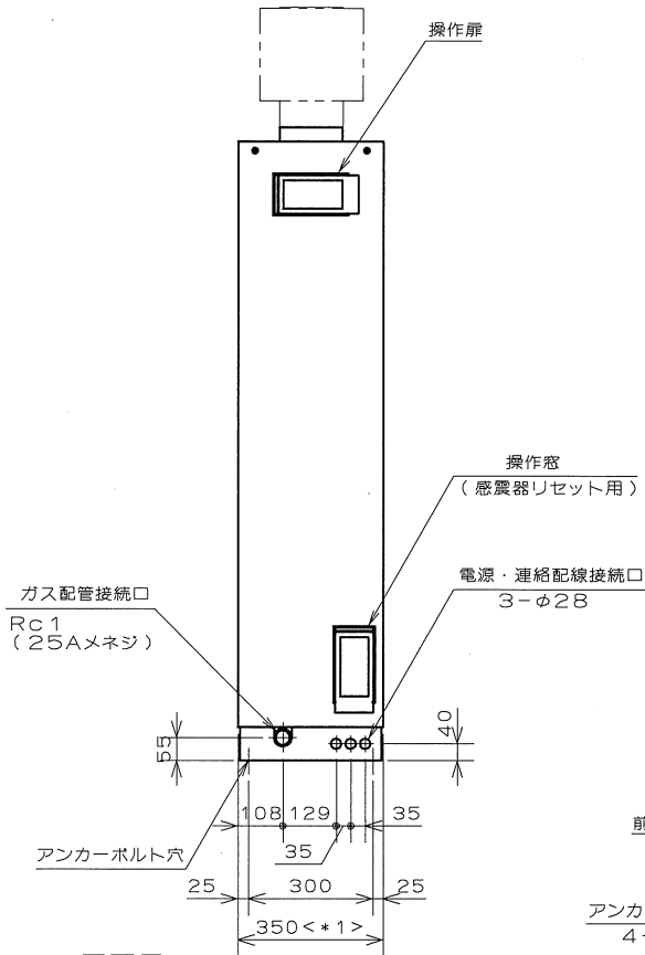
正面図
