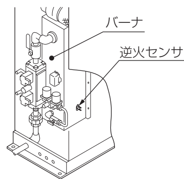
逆火センサ
