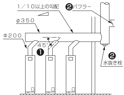
3台設置の場合
