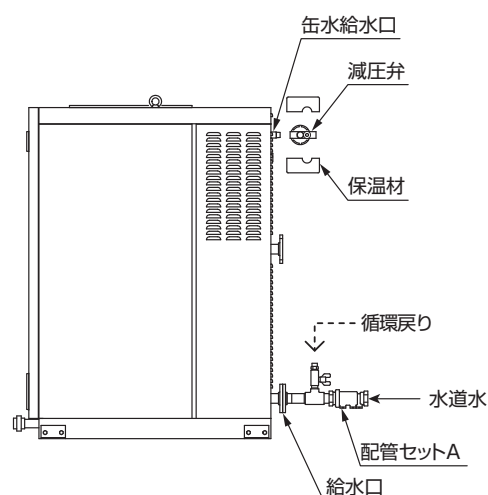
水道直結・給湯循環式
