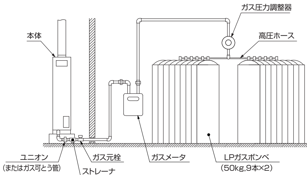
設置例 (調整器：自動、気温：5°Cの場合)
