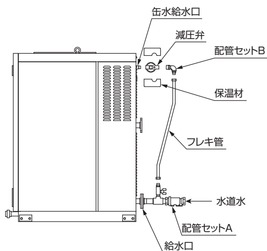
水道直結・給湯先止め式
