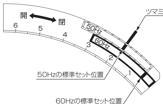
指定の位置にツマミをあわせる
