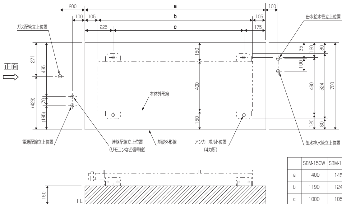
基礎参考図
