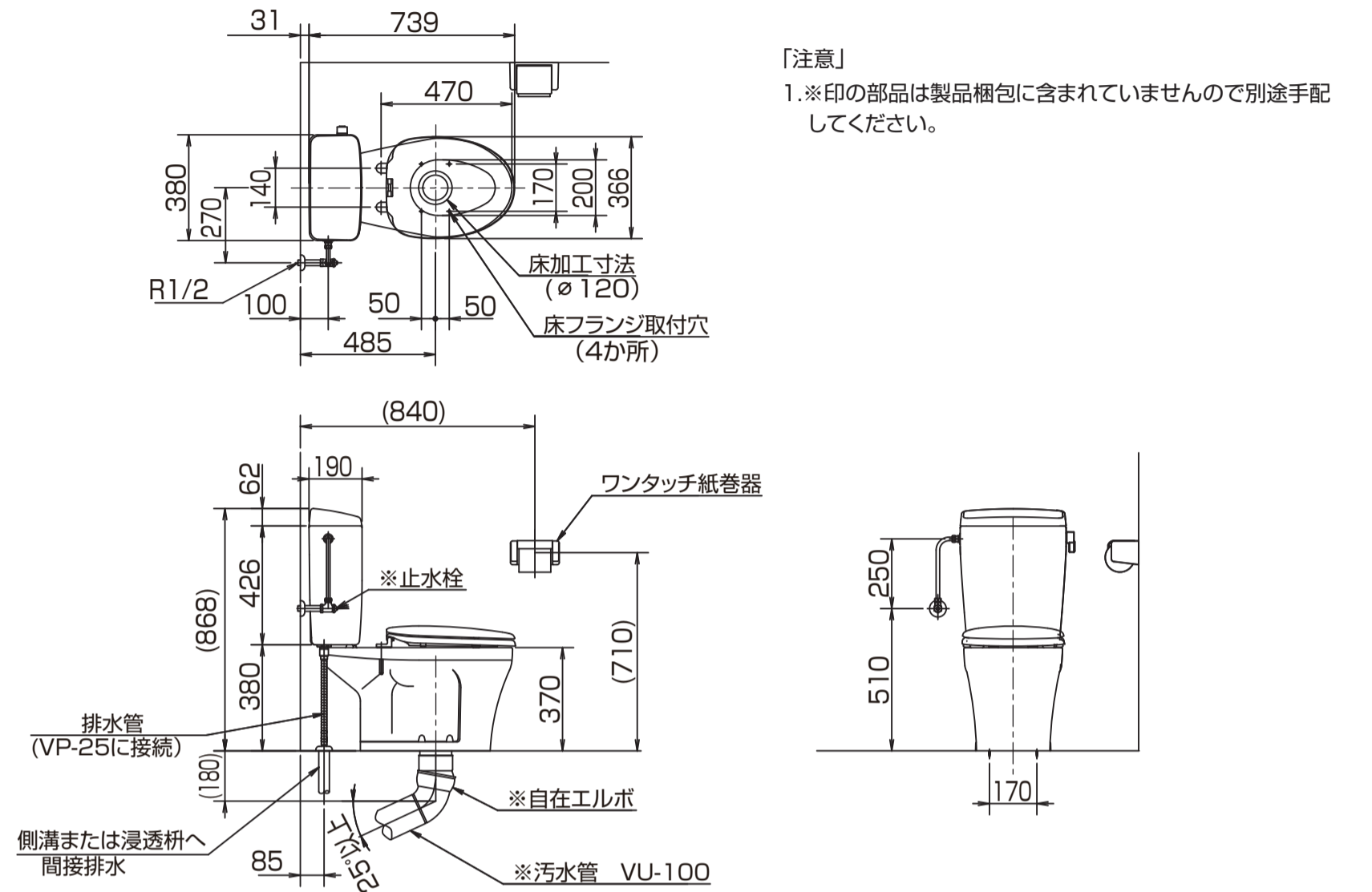
施工寸法図 ATW-50
