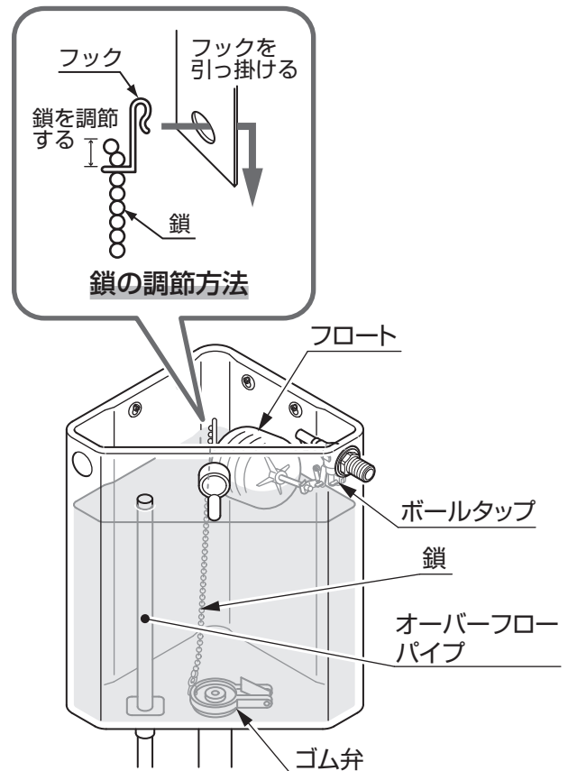
給水タンク内部
