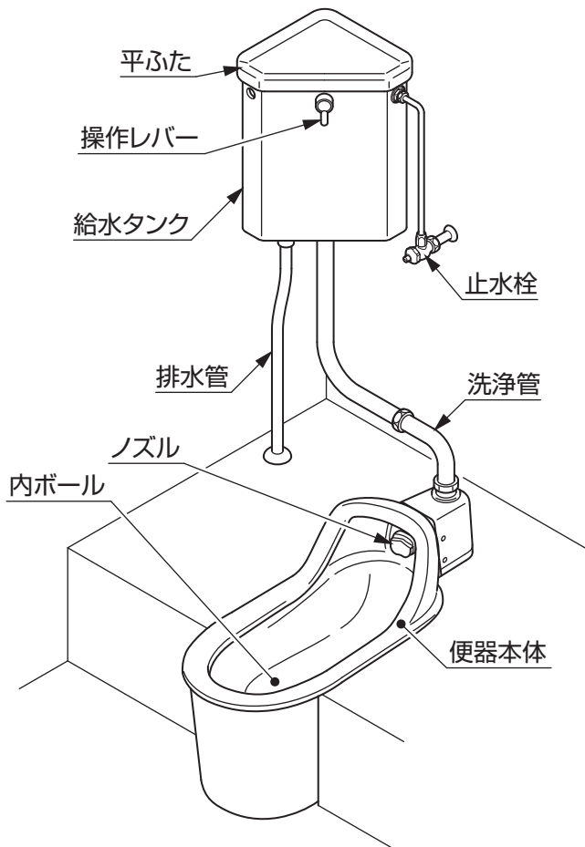
外観図 例：(タイプなし)
