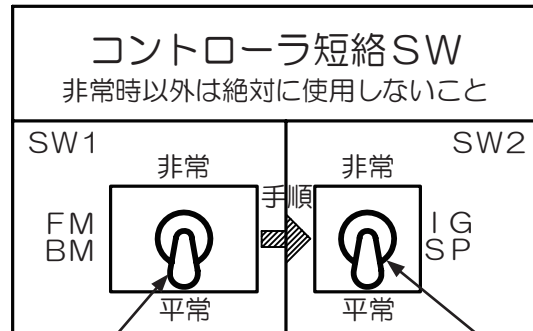
SW1 送風機およびバーナ送風機の短絡スイッチです
