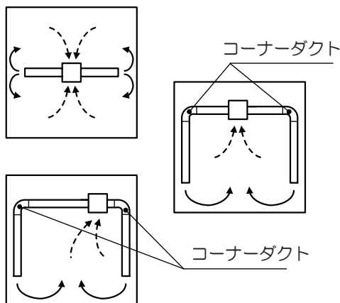
正方形ハウスの場合
